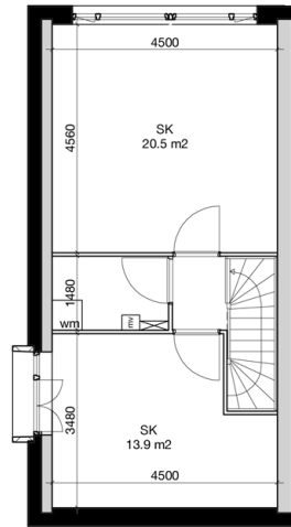
2e verdieping - optie
