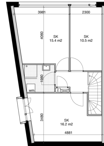
2e verdieping - optie
