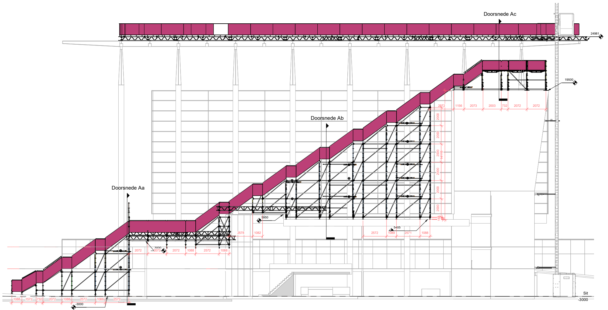
Aanzicht
