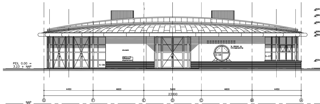
noordgevel
