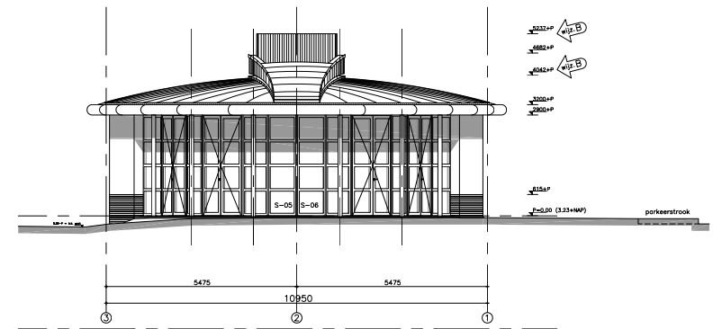
oostgevel
