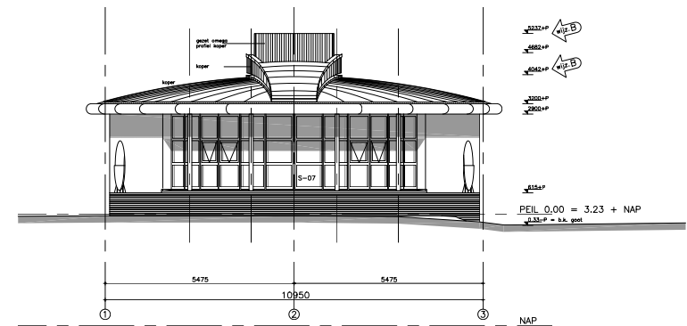
westgevel
