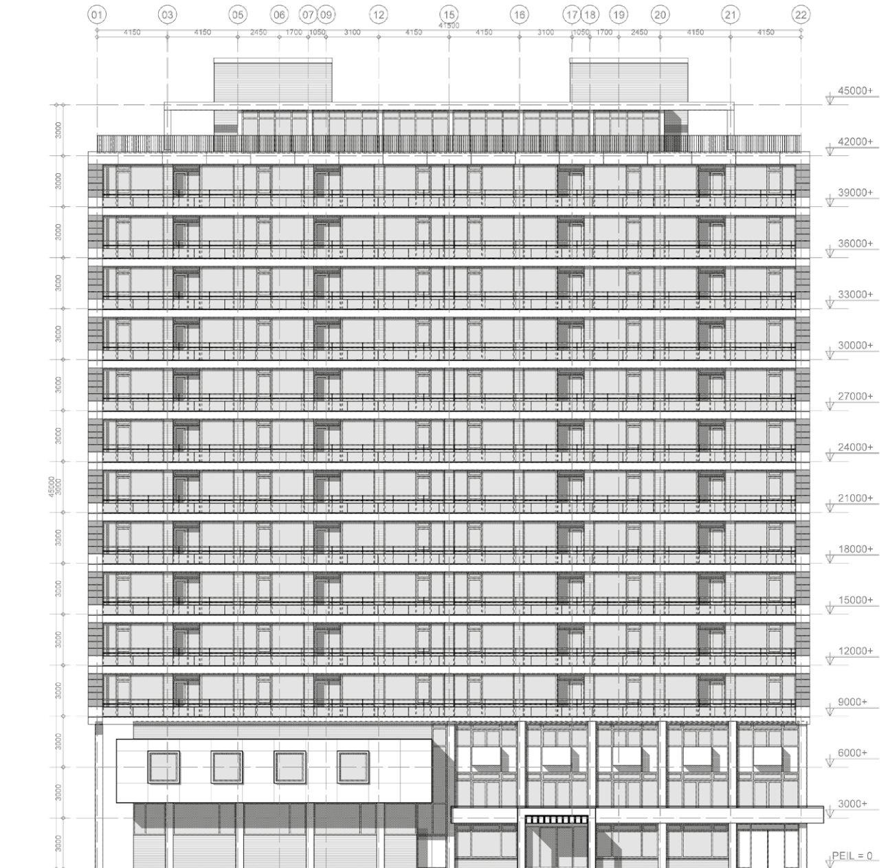
Voorgevel
