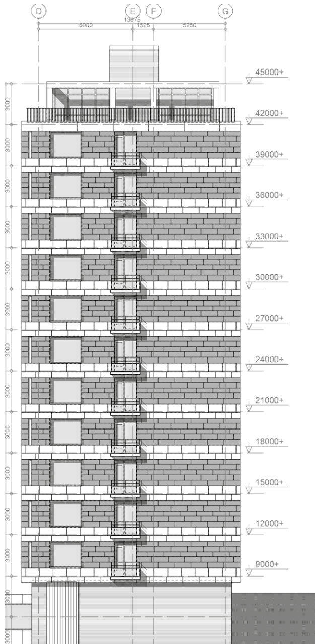
Rechter zijgevel
